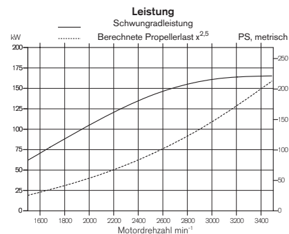
D4-225 mit HS45AE Wendegetriebe
